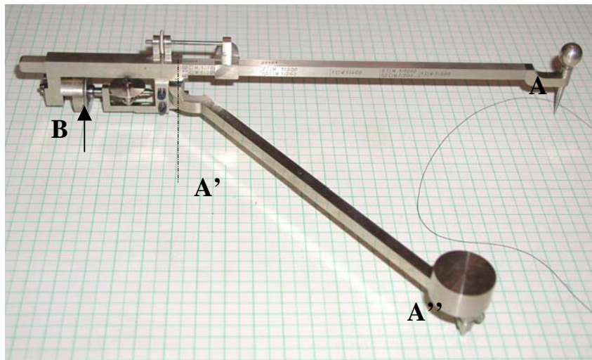
12 : Planimètre polaire Amsler, vers 1877, coll. SS n°340.
