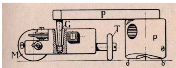
14 : Assemblage du bras polaire dans un planimètre compensateur (extrait de li. Le pôle A' du bras A'A' est un stylet ; sa pointe fixe est son centre de rotation. A' est un axe d'assemblage ou une rotule destinée à reposer sur le fond d'une cuvette sur le bras porteur.
